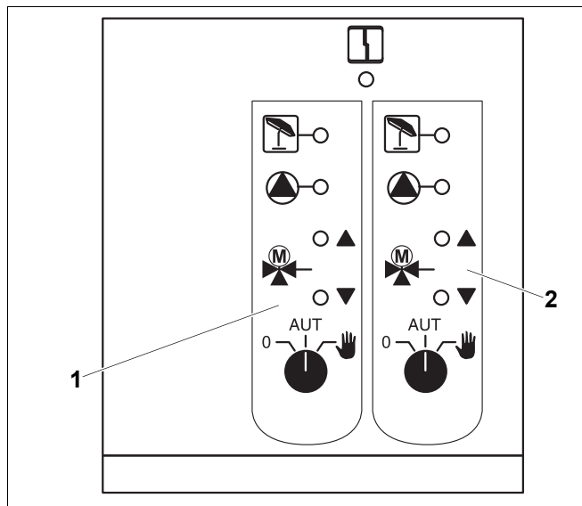
Рис. 25 Функциональный модуль FM442
