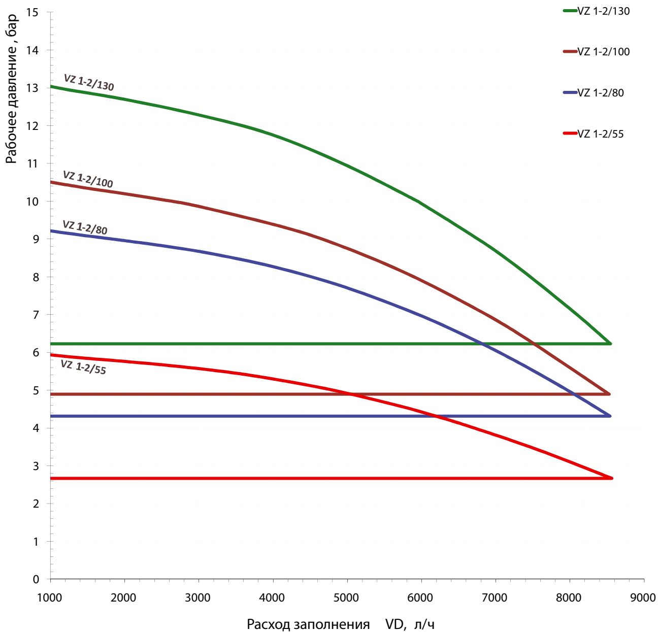
Насосные установки с функцией заполнения Variomat VZ
