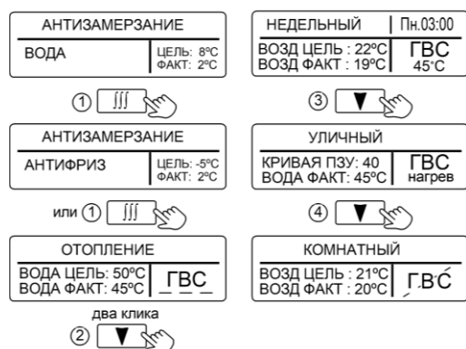
Рисунок 5. Режимы работы прибора
