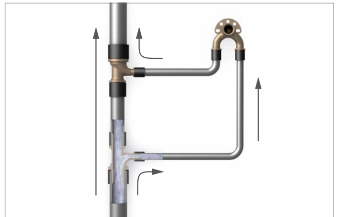
Рис. 5-5. Принцип работы кольцевого трубопровода с изогнутой Т- образной трубкой RAUTITAN RX+
