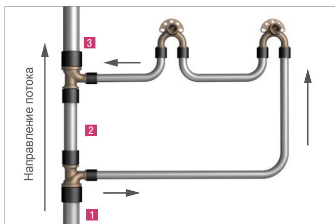
Рис. 5-9. Принцип работы кольцевого трубопровода с изогнутыми Т-образными трубами RAUTITAN RX+
