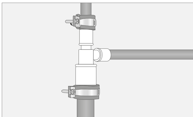
Рис. 34-1 Формирование неподвижных опор с хомутами
