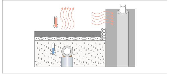
Рис. 37-5 Прокладка под горячим асфальтобетонным покрытием
